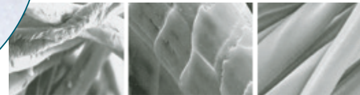
Die Faseroberfläche von Baumwolle, Wolle und Tencel im Vergleich.
